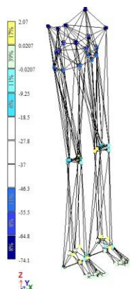
Рисунок 2 – Значення горизонтальних складових переміщень вузлів моделі нижньої частини ОРА людини уздовж координатної осі Oх (мм)
