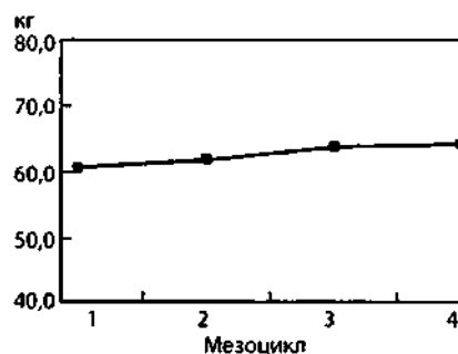
РИСУНОК 2 – Абсолютная интенсивность (кг) тренировочной нагрузки у тяжелоатлетов 16–18 лет с учетом различий по весовым категориям в разных мезоциклах годового макроцикла: 1 – втягивающий; 2 – базовый; 3 – контрольно-подготовительный; 4 – соревновательный; ▲ – первая группа; ■ – вторая группа; ○ – третья группа
